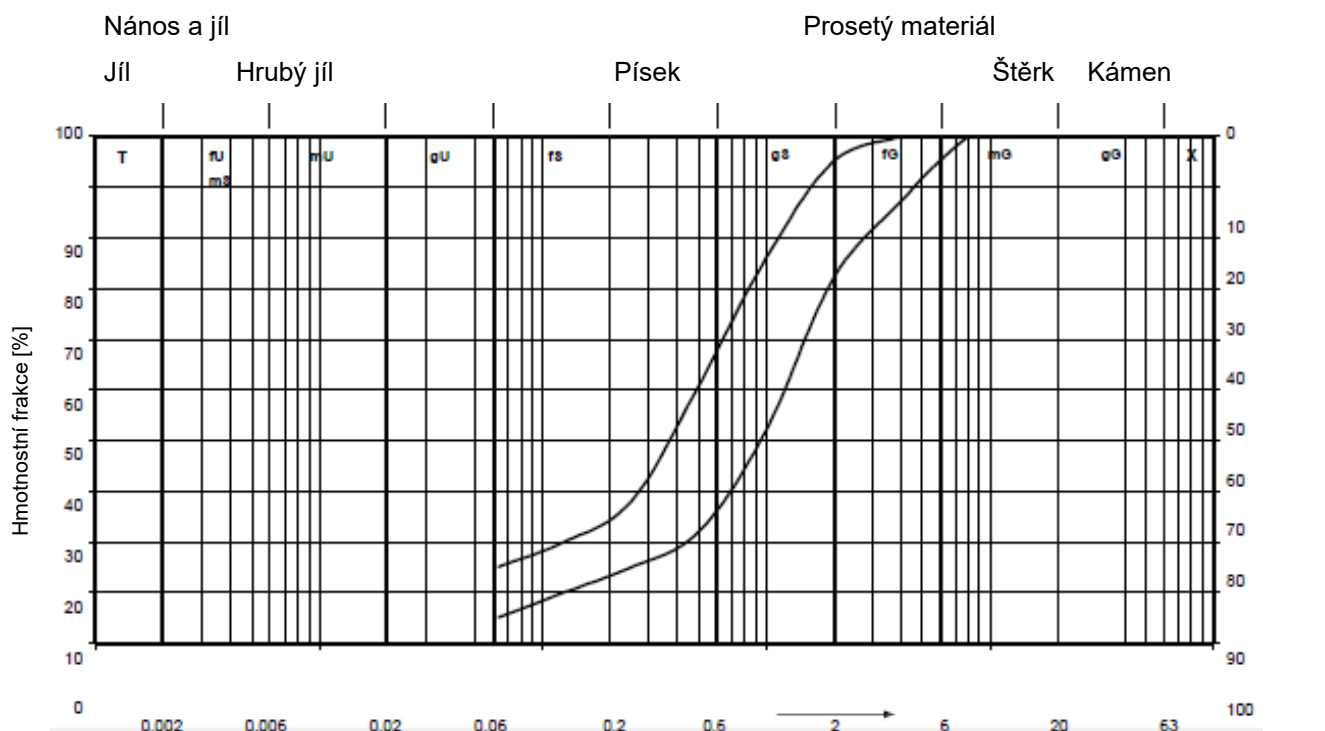
Obrázek č. 9: Doporučená křivka zrnitosti pro podkladové vrstvy vegetace (zásypového materiálu u zatravněných povrchů; směs by se měla nacházet v dolní části křivky doporučeného rozmezí zrnitosti, avšak požadavky na funkčnost směsi mají v takovém případě přednost)
